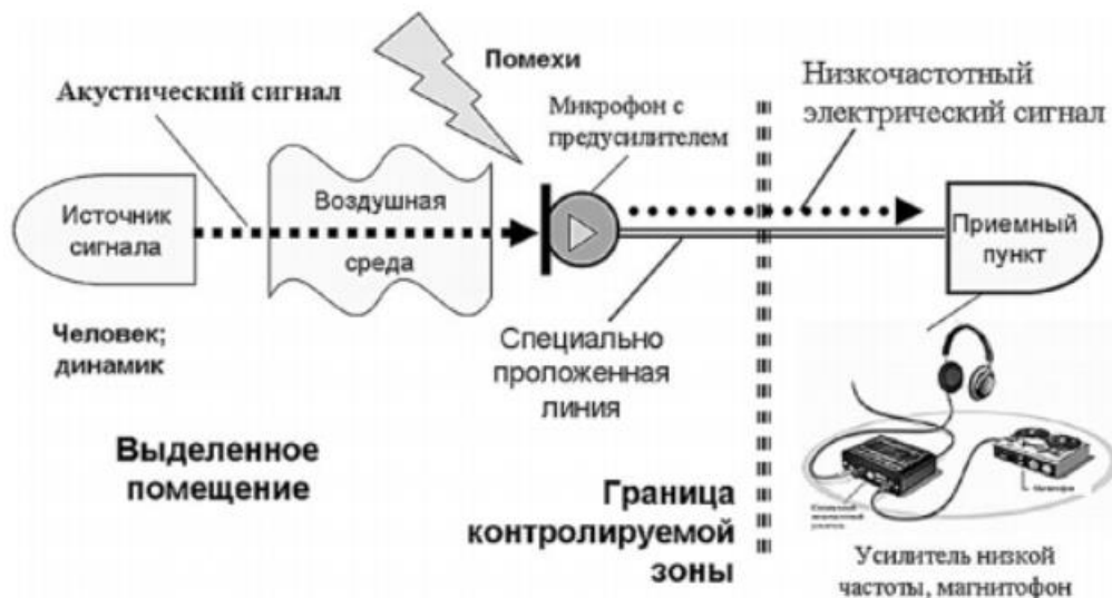
Рисунок 3 - Перехват речевой информации с помощью диктофона
