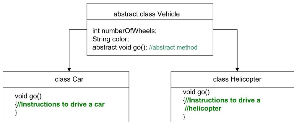
Рисунок 6.1. Иерархия классов
