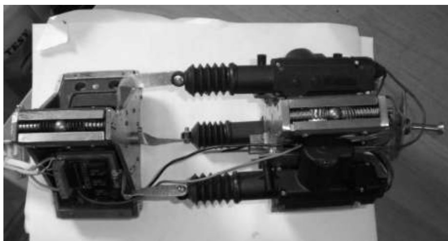
Рис.5. Фото собранного червеподобного робота с двумя модулями и электрическими приводами (прототип устройства)
