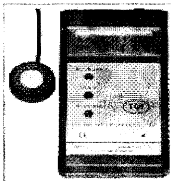
Рисунок 1 - Внешний вид прибора ТКА-ПКМ-08.
