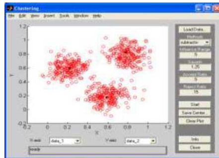
Рисунок 10. Результат работы программы Clustering (центры кластеров окрашены в черный цвет)
