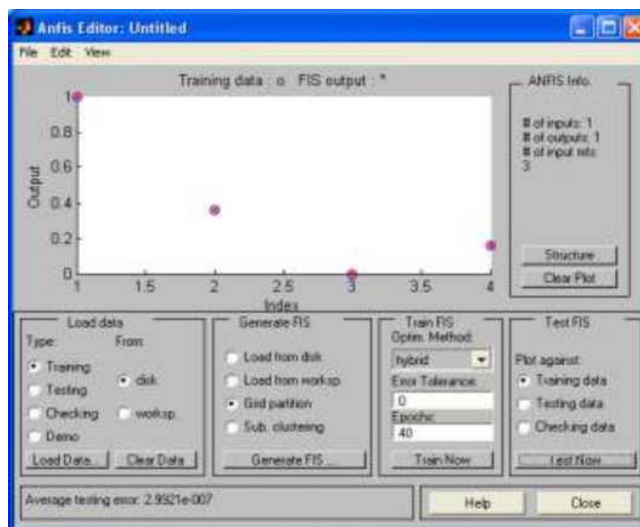
Рисунок 9. Результат тестирования обученной системы
