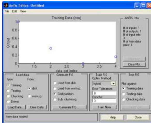
Рисунок 5 - Окно редактора после загрузки обучающей выборки
