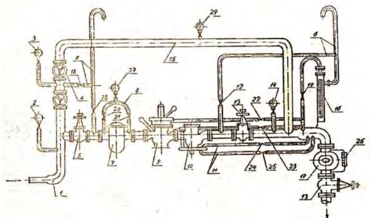
Рис. 6. Схема ГРП:
