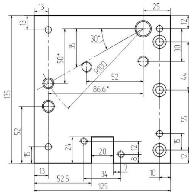
Рис. 1 – Эскиз детали
