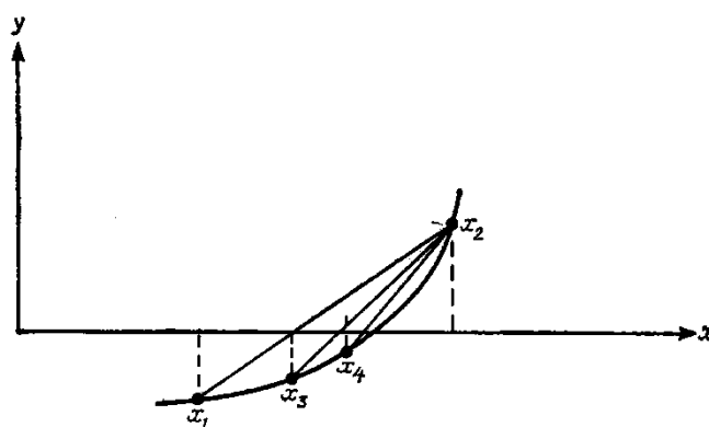
Рис. 5. Метод хорд
