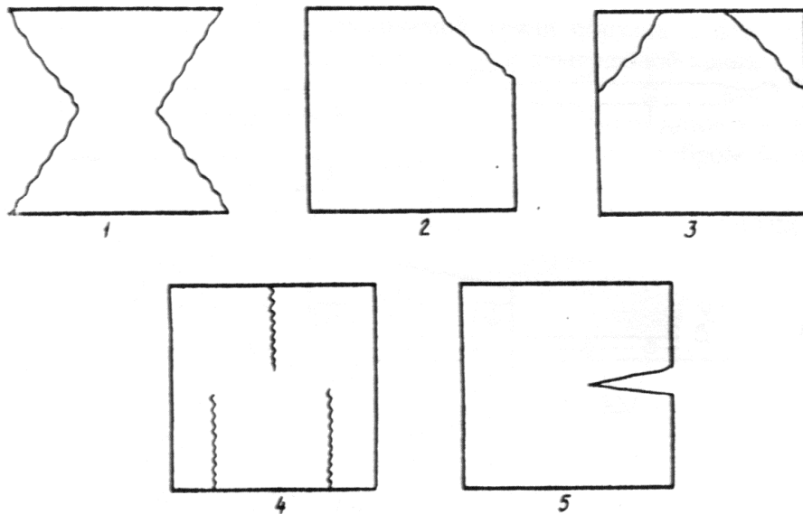
Рисунок 6 – Характер разрушений при проведении испытаний образцов-кубов на осевое сжатие: 1 – нормальное разрушение; 2-5 – дефектные разрушения
