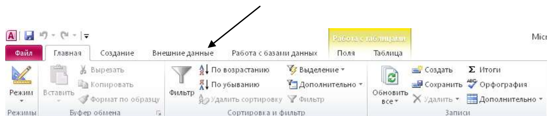
Рис.5 – Кнопка «Фильтр»
