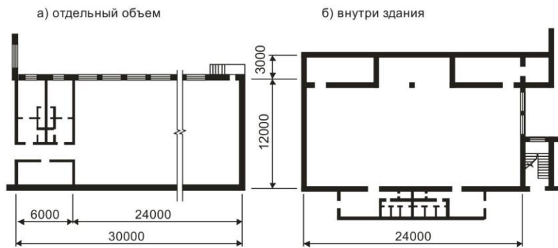
Рис. 4. Пример компоновки спортивного зала
