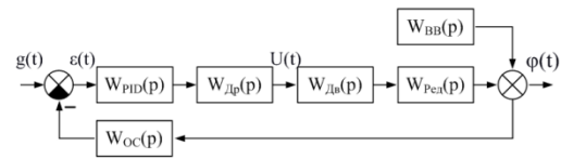
Структурная схема одного канала САУ
