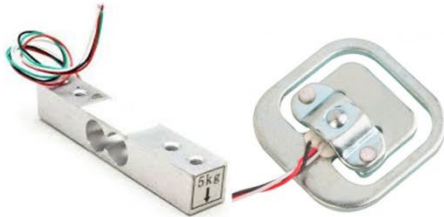
Тензодатчики для измерительных манжет и для стопы
