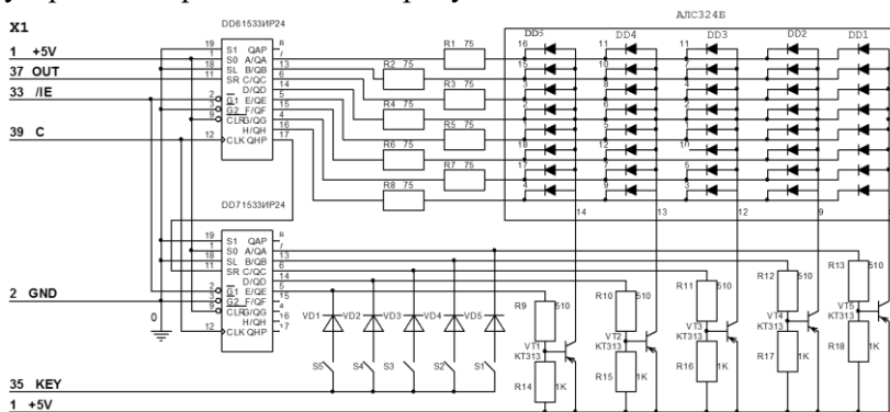
Рисунок 8-Схема устройства динамической индикации.
