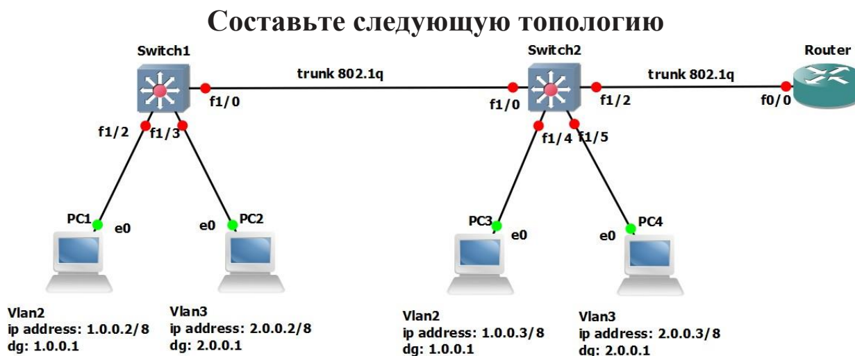
Рисунок 4 – Исследуемая сеть
