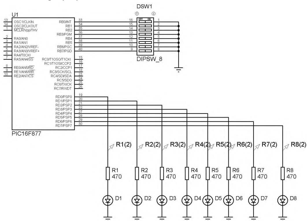
Рисунок 1 – Схема включения
