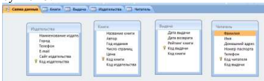
Рис.25 – База данных после редактирования
