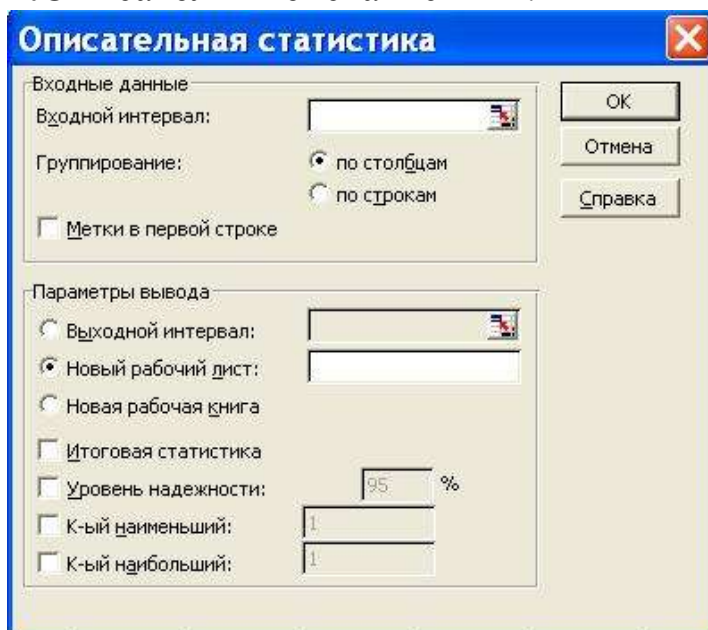
Рис. 14 - Диалоговое окно инструмента Описательная Статистика
