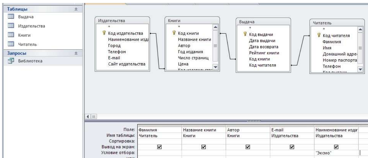
Рис. 40 – Окно запроса с условием
