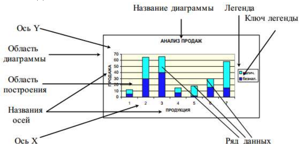
Рис. 5 - Основные компоненты диаграммы
