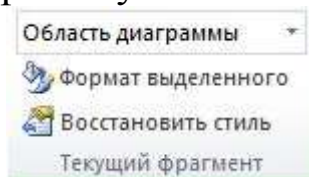
Рис. 11 - Окно области диаграммы
