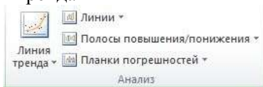
Рис. 12 - Окно линии тренда
