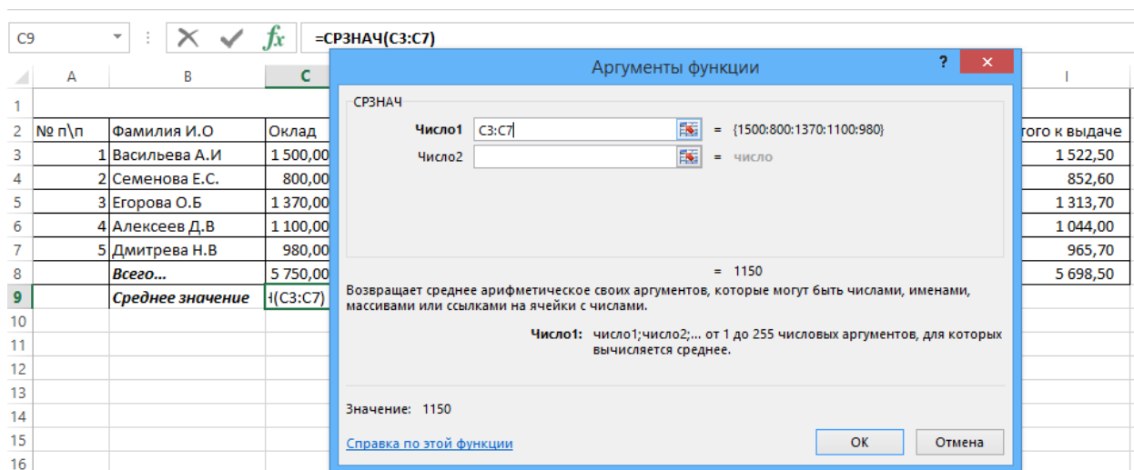
Рис. 4 - Окно мастера функций
