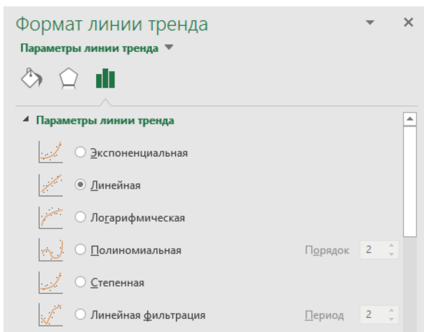
Рис. 13 Диалоговое окно линии тренда
