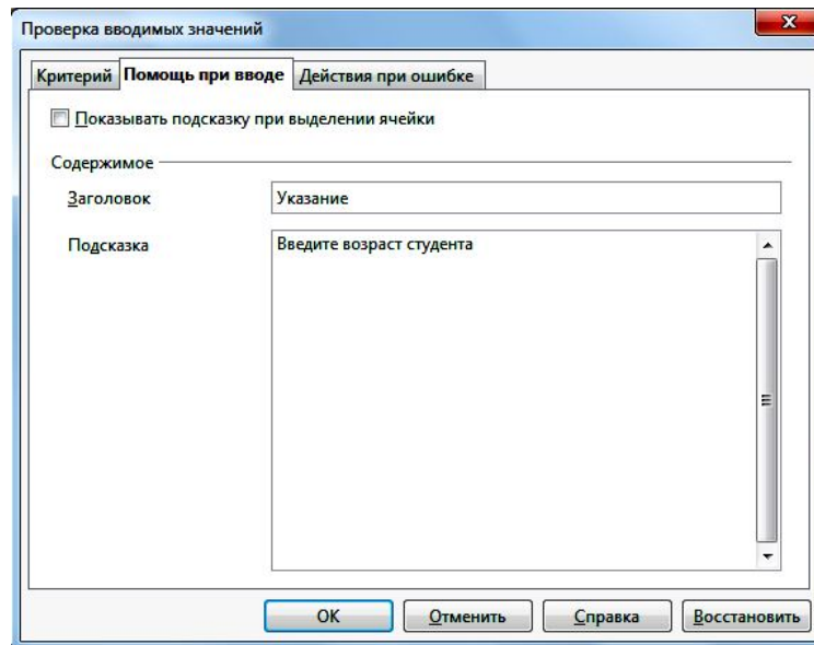
Рис. 49. Установка подсказки для проверки вводимых значений в базу данных
