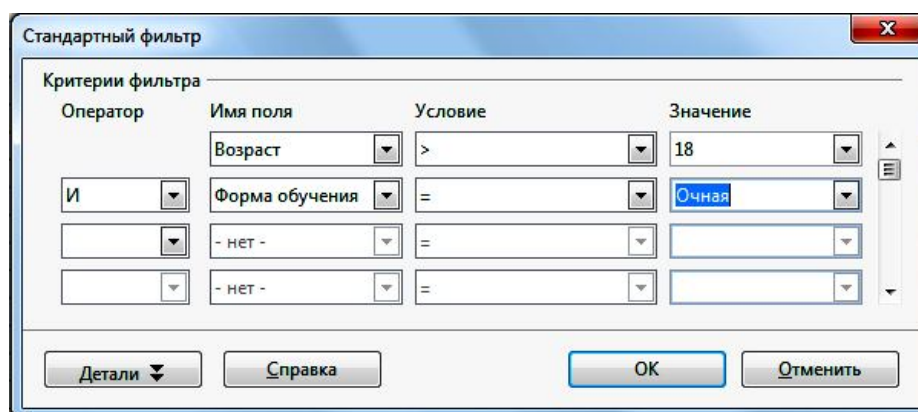
Рис. 56. Стандартный фильтр
