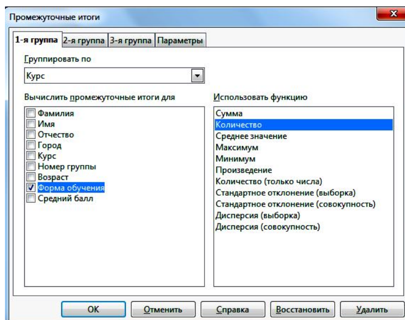
Рис. 58. Промежуточные итоги
