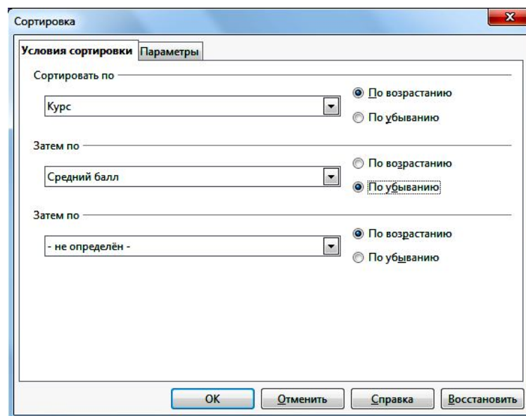
Рис. 54. Сортировка данных
