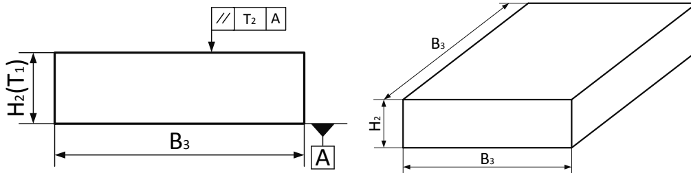
рис. 4 Требования к точности обработанной детали (а) и образец-изделие (б)
