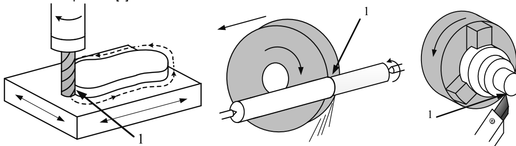
рис. 1 Примеры функциональных точек по ISO 230-1:2012
