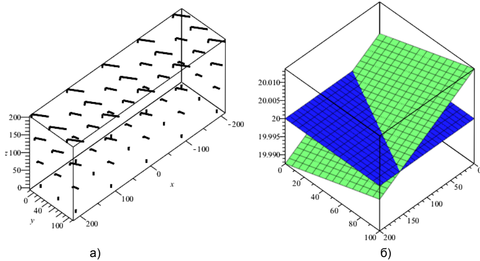
рис. 3 Векторный баланс точности плоскошлифовального станка (а), номинальная и реальная обработанные поверхности (б)
