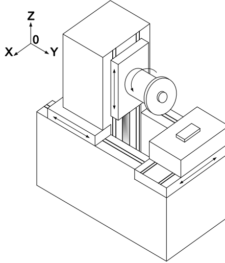
рис. 2 Формообразующая система плоскошлифовального станка (адаптировано из [9])
