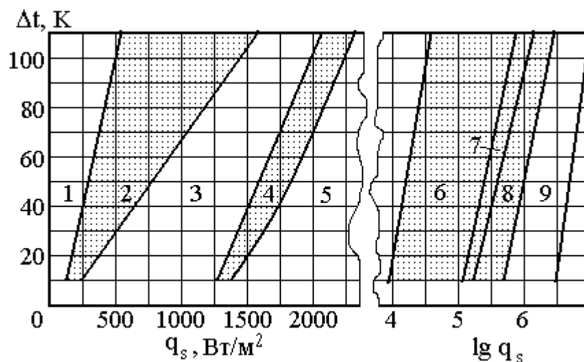
Рисунок 2 - Диаграмма выбора способа охлаждения: 1 – естественное воздушное; 2 – естественное и принудительное воздушное; 3 – принудительное воздушное; 4 – принудительное воздушное и жидкостное; 5 - принудительное жидкостное; 6 – принудительное жидкостное и естественное испарительное; 7 – принудительное жидкостное, принудительное и естественное испарительное; 8 – естественное и принудительное испарительное; 9 – принудительное испарительное
