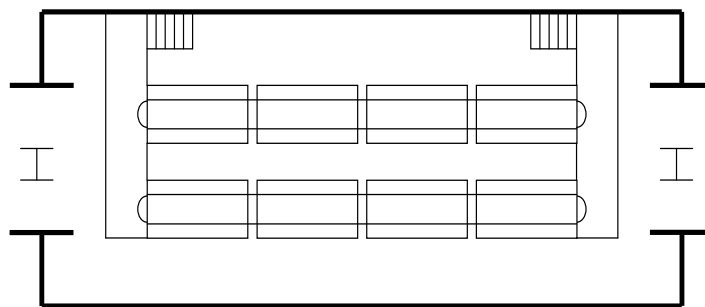
Рисунок 3– Схема планировки зоны ТО при прямом расположении постов
