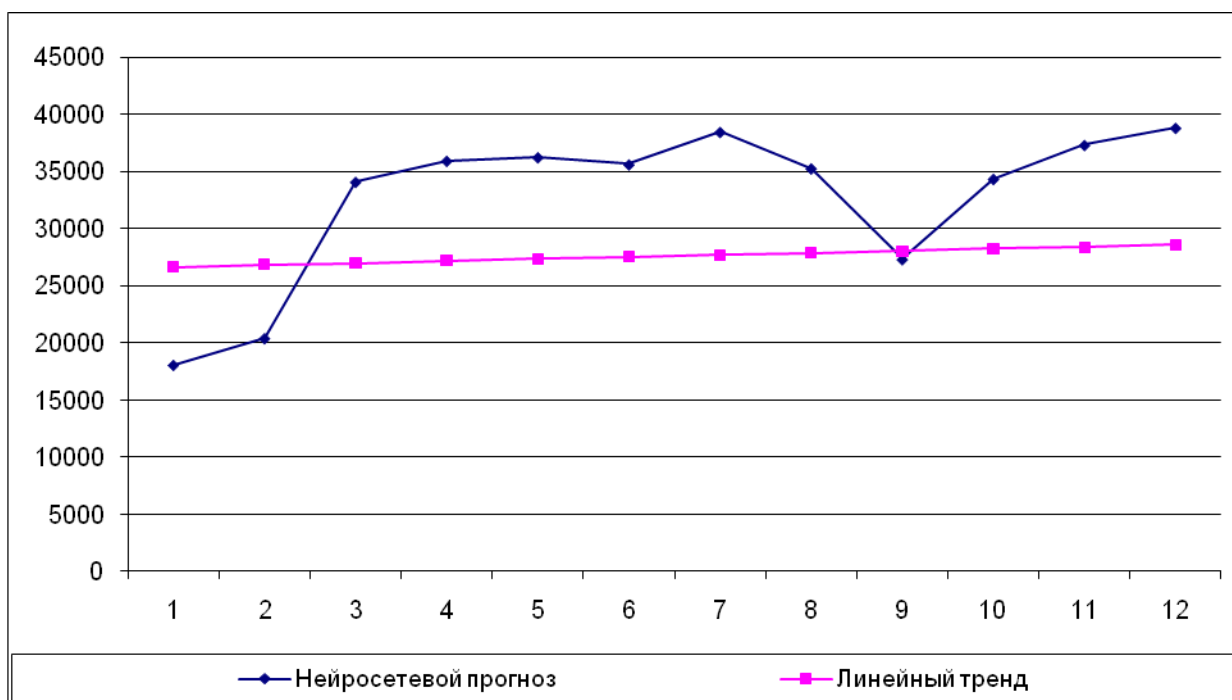
Рисунок 42 - Результаты прогнозов выручки на 2006 год нейросетью и по линейному тренду
