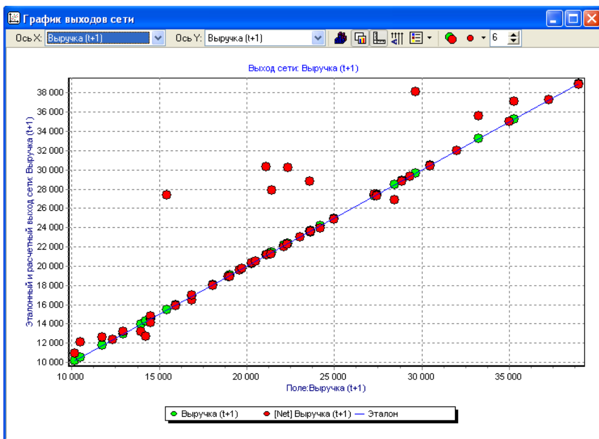
Рисунок 37 - Эталонный и расчетный выход сети по показателям: фактическая и прогнозируемая выручка в период 2001-2004 гг.
