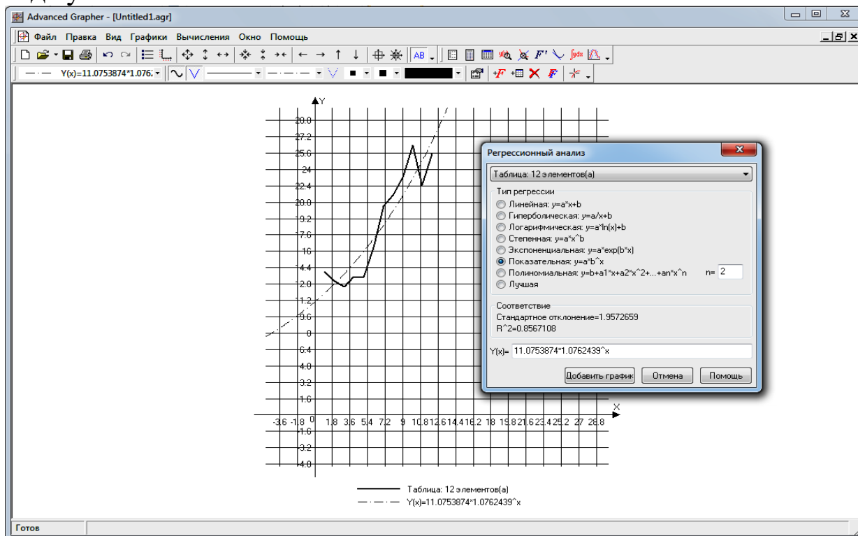
Рисунок 12 – Аппроксимация зависимости показателя выпуска продукции от времени показательной функцией
