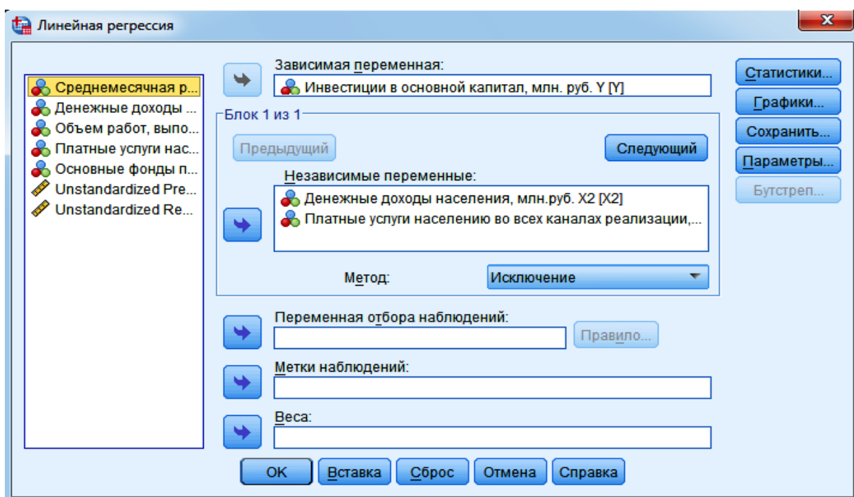
Рисунок 23 – Линейная регрессия
