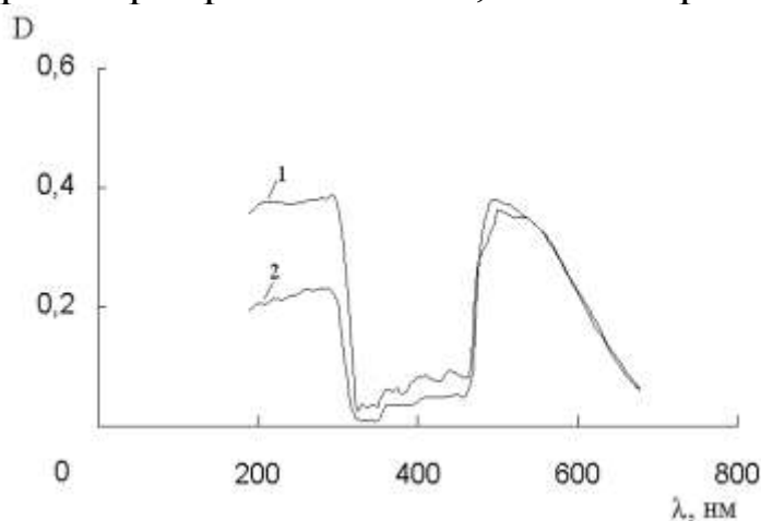
Рисунок 1 – Спектры поглощения салицилата железа
