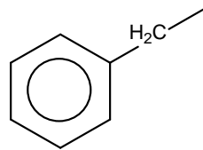
бензил
