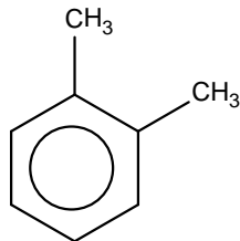
o - (ортоксилол)
