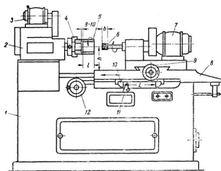
Внутришлифовальный станок
