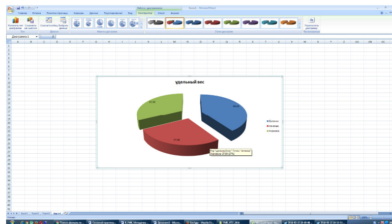
Рисунок 3 – Круговая диаграмма
