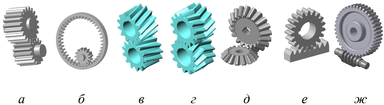
Рис. 2. Типы зубчатых передач:
