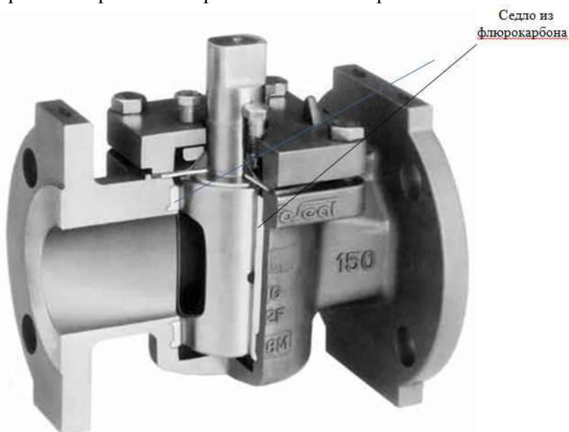
Рис.3.2 Кран пробковый
