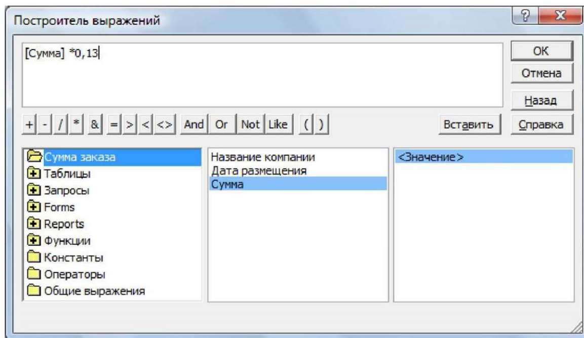
Рисунок 2.8 - Построитель выражений
