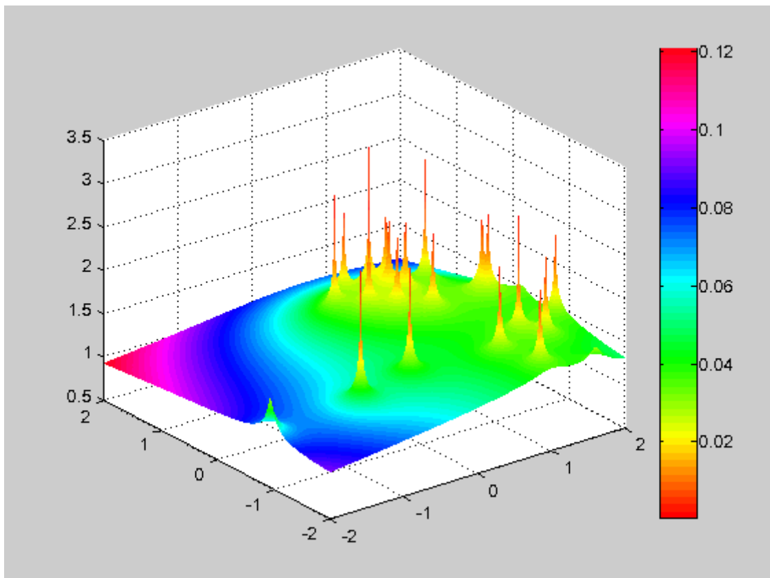
Рисунок 21 - Логарифм потенциала
