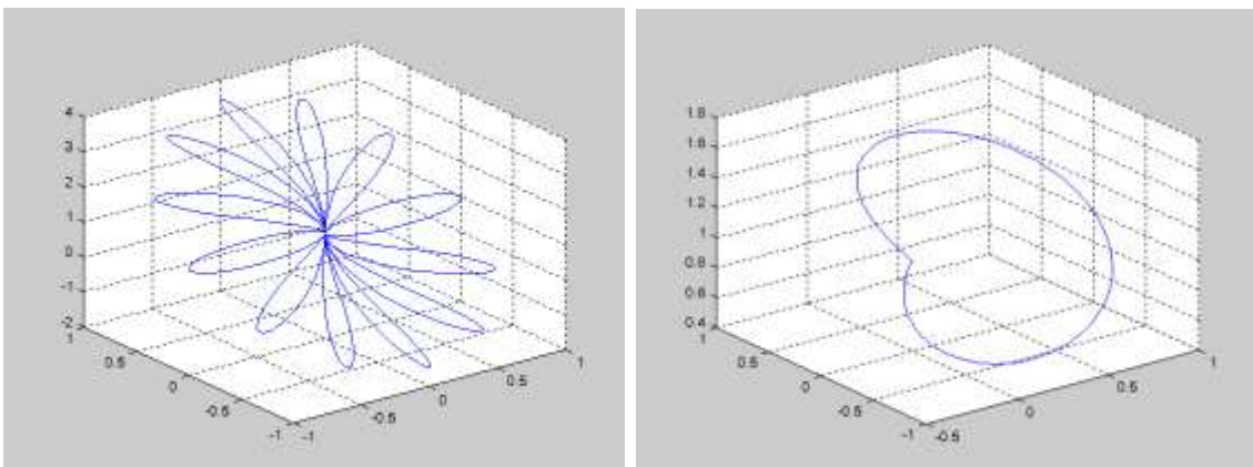
Рисунок 22 – Пример графиков
