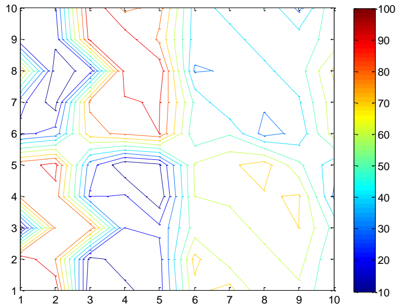
Рисунок 1 – Расшифровка цветов
