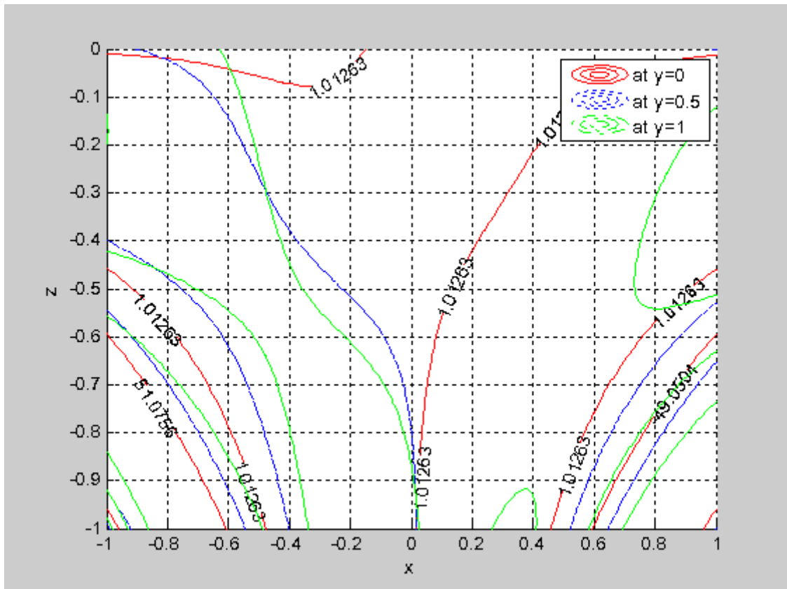
Рисунок 28 - Линии уровня лапласиана рабочей функции
