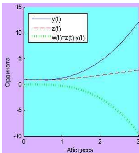
Рисунок 11 – Итоговый график
