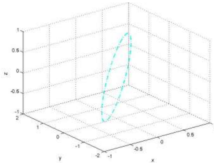
Рисунок 8 – Координатная кривая
