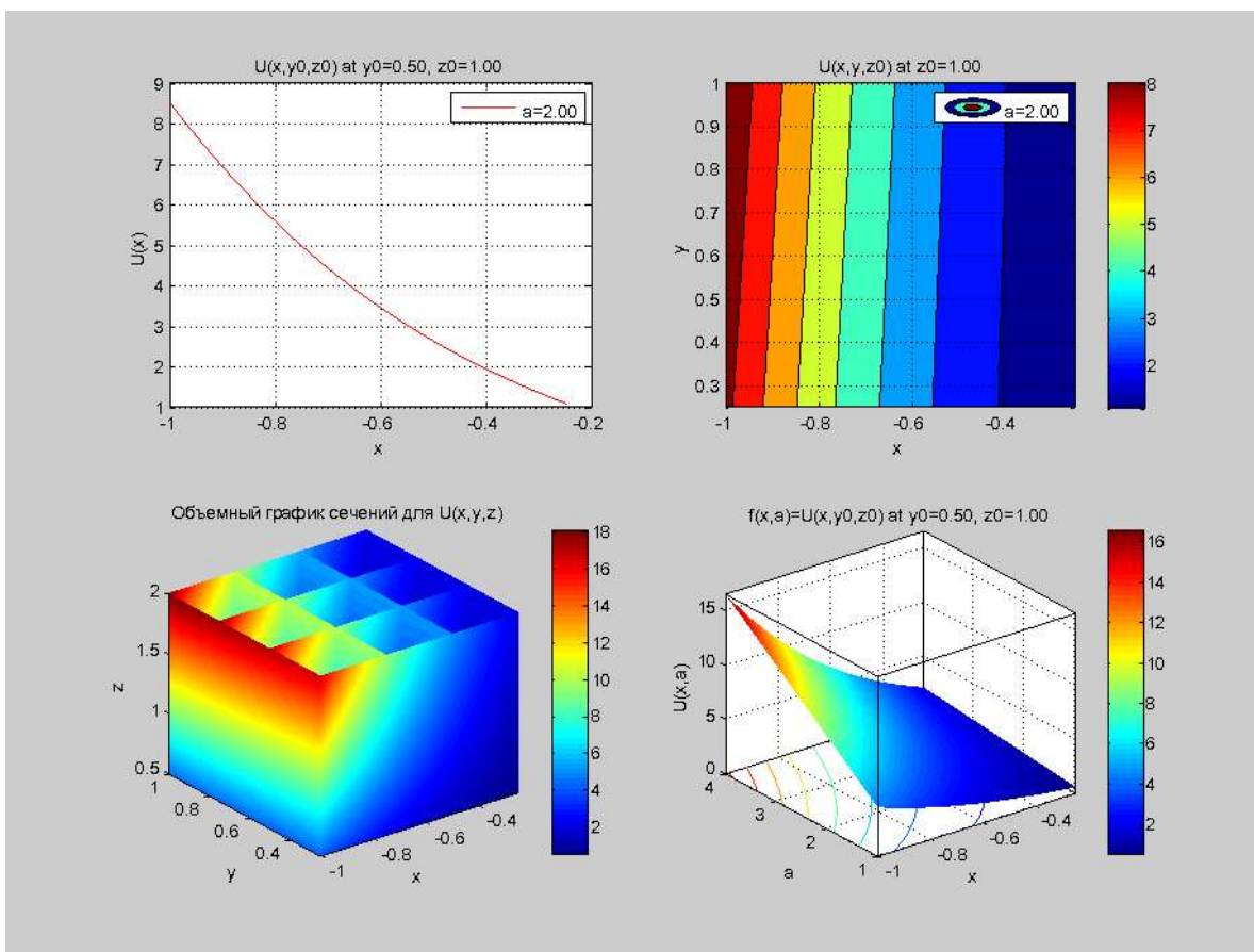
Рисунок 29 – 3-D график функции
