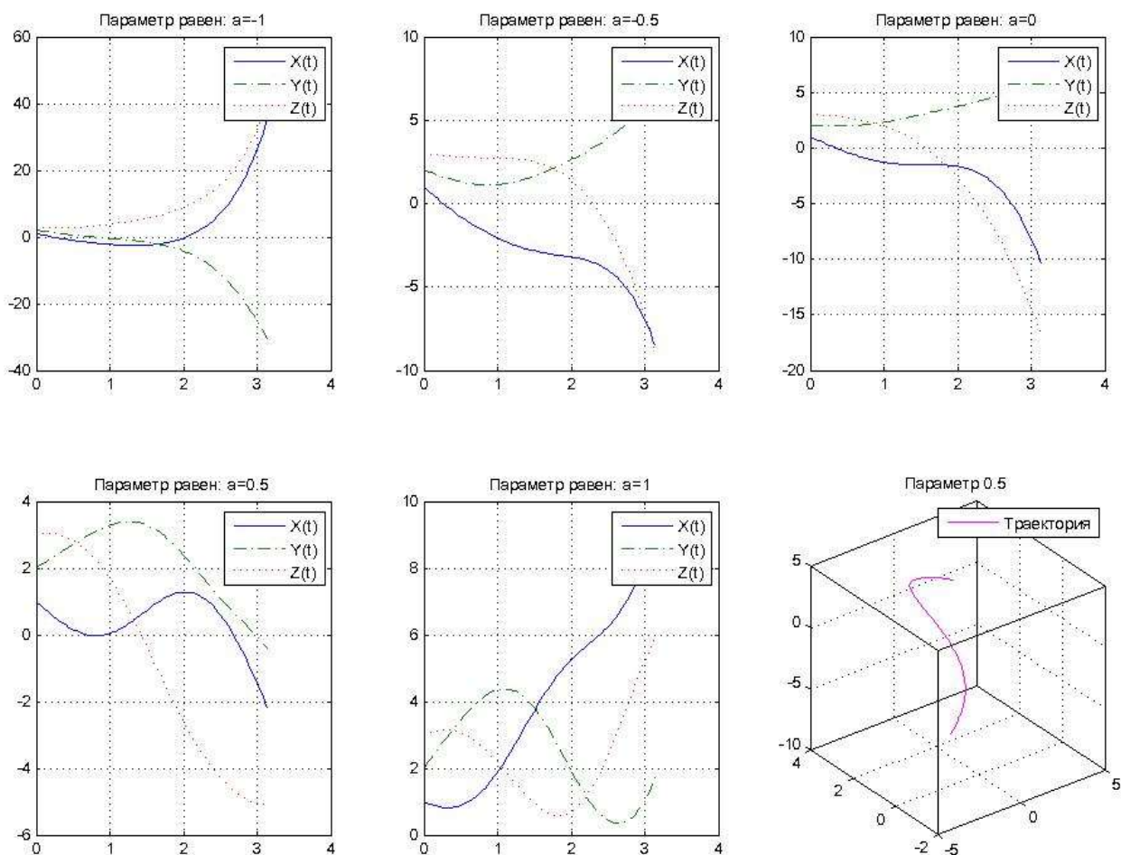
Рисунок 16 – Семейство решений
