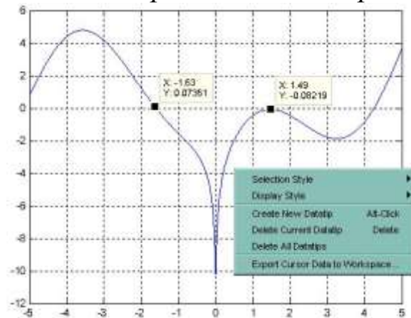
Рисунок 15 – Отрезок x * \cos(x) + \ln(x^2) = A
