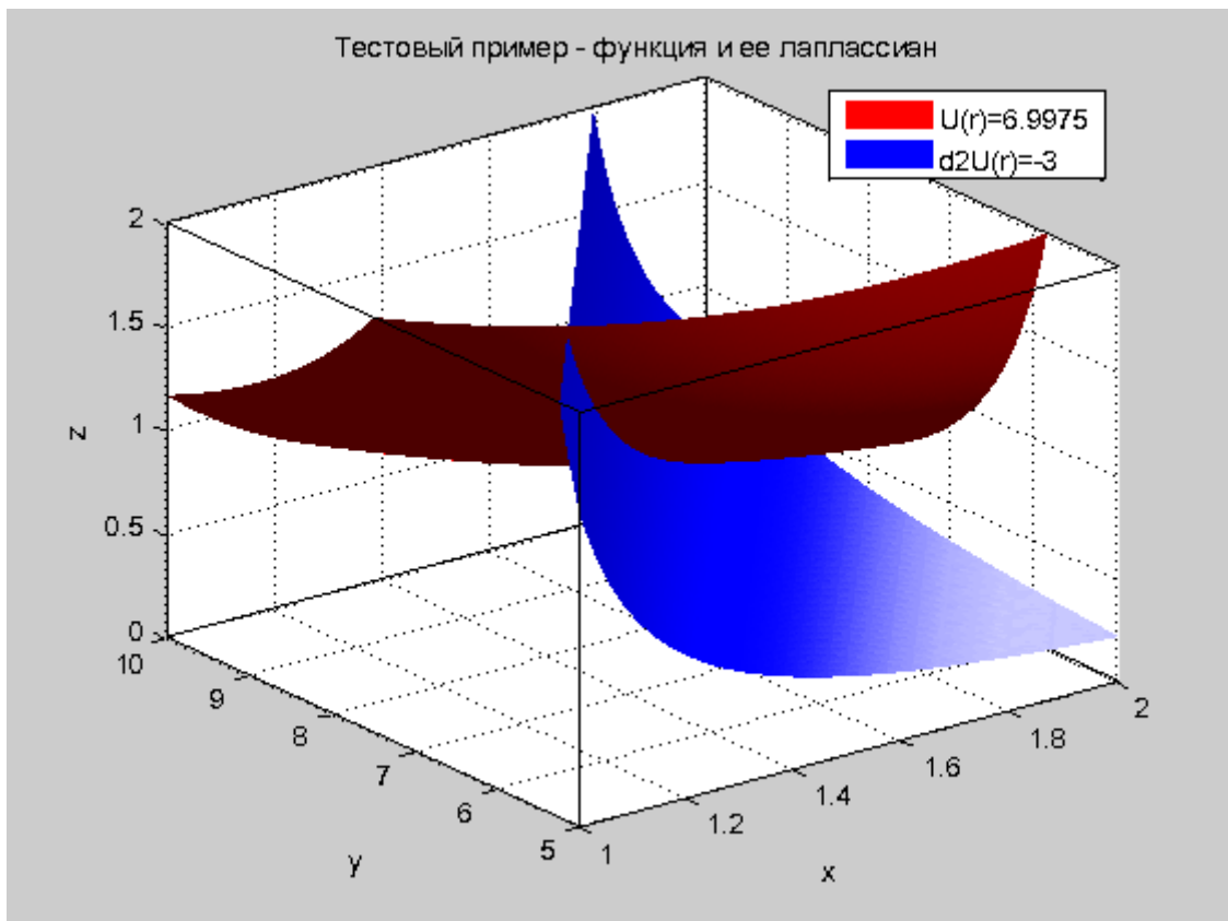
Рисунок 24 – Тестовая функция
