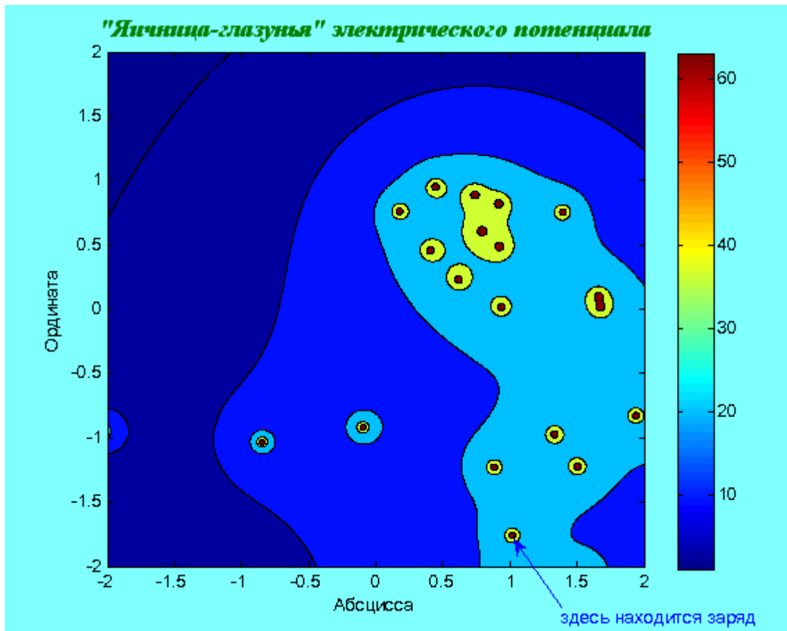
Рисунок 19 – «Яичница-глазунья» электрического потенциала
