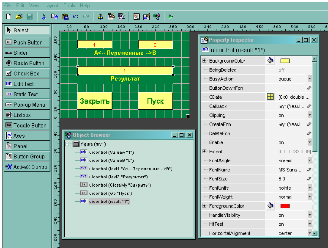
Рисунок 17 - Простейший пример GUI-программы
