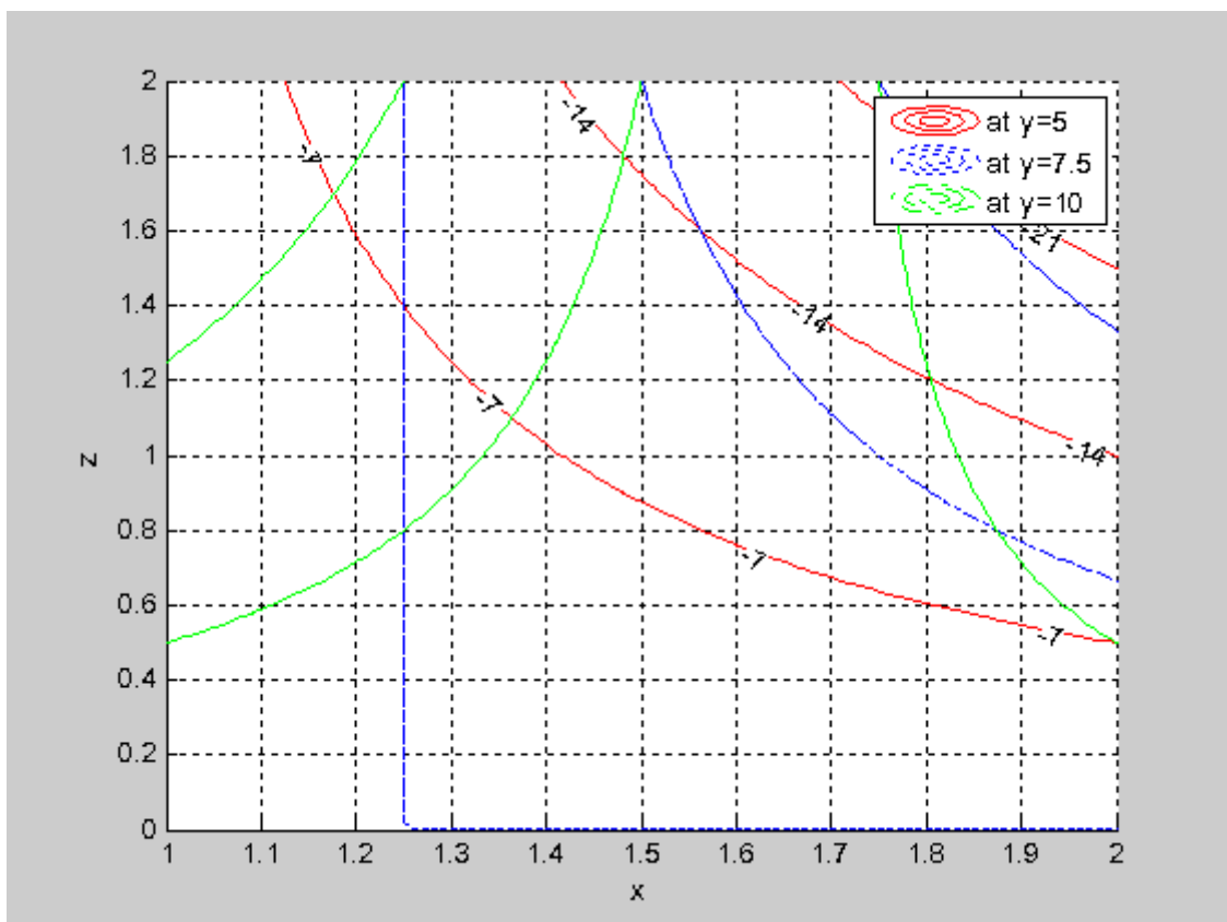
Рисунок 25 – Линии уровня лапласиана тестовой функции
