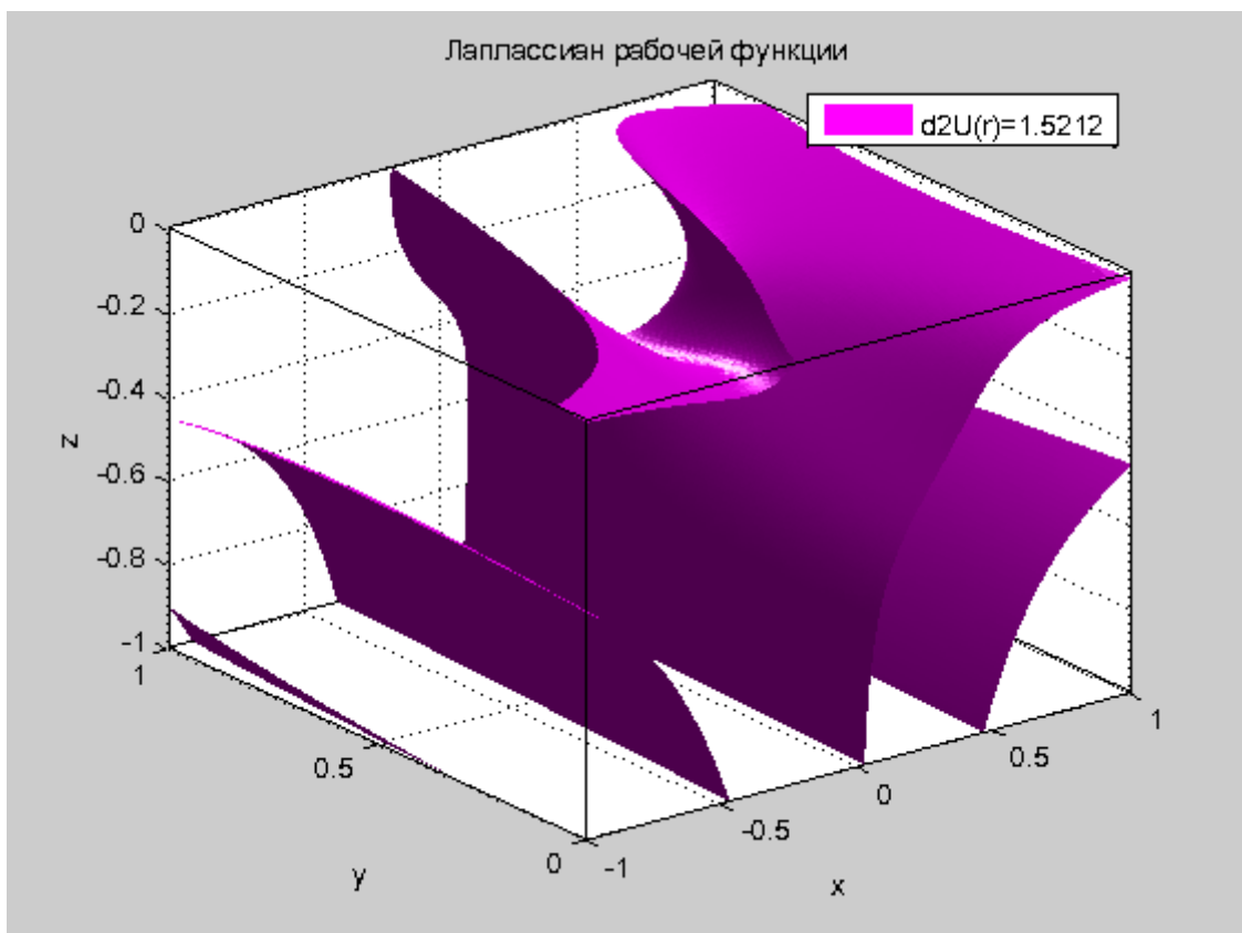
Рисунок 27 – Лапласиан рабочей функции
