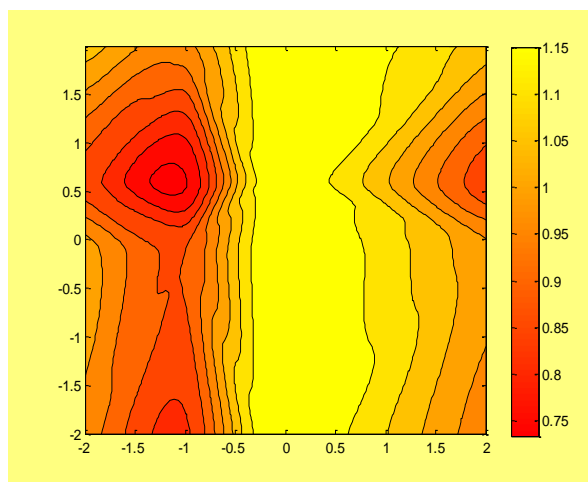
Рисунок 5 – первоначальная сетка
