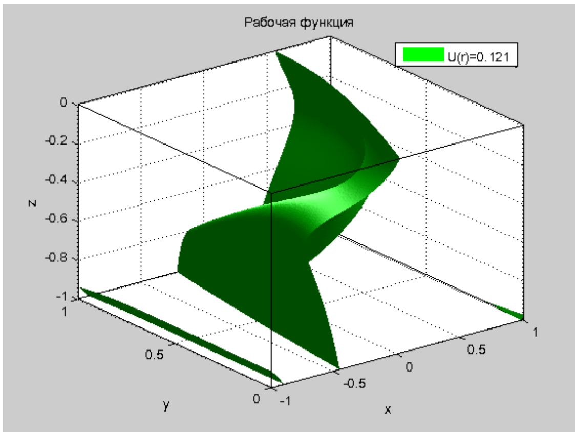
Рисунок 26 – Рабочая функция
