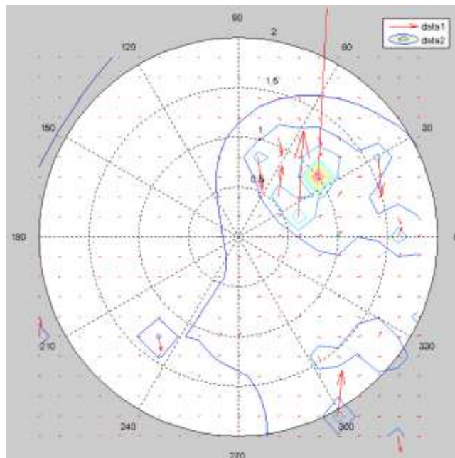
Рисунок 20 - График скоростей, напряженностей и потенциала
