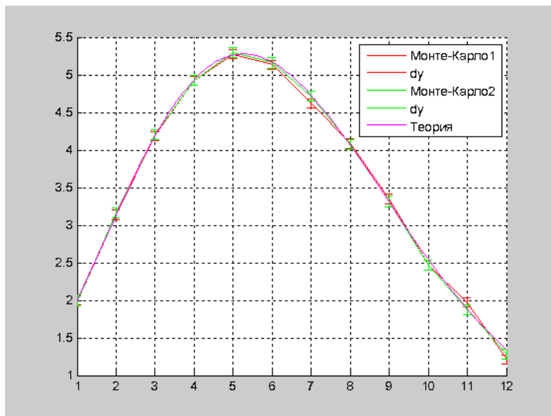
Рисунок 23 – Группы итераций
