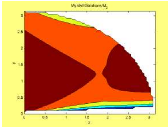
Рисунок 13 – Проверочный график
