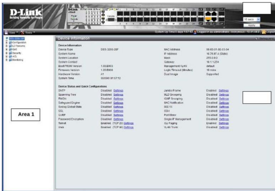
Рисунок 2 – Страница управления
