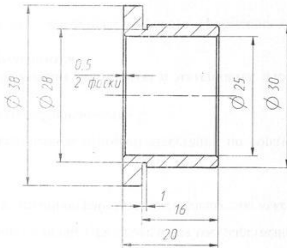
Рис.3. Подшипник.
