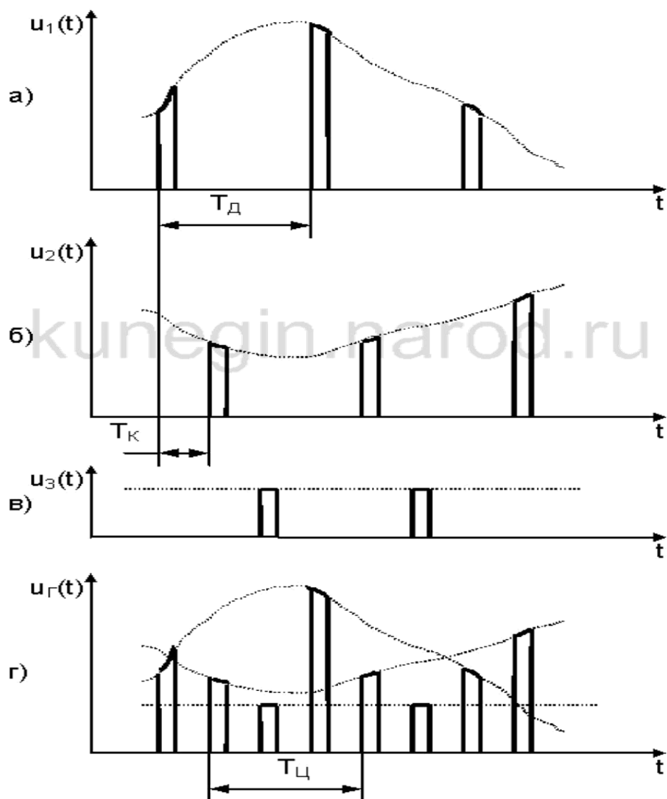
Рисунок 1 – Диаграмма временного уплотнения дискретизированных АИМ-сигналов
