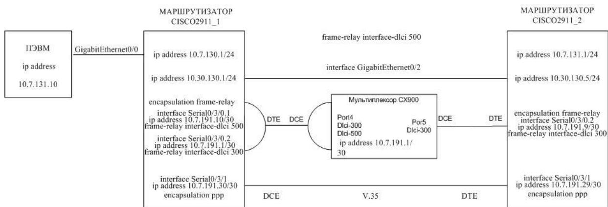
Рисунок 6 – Фрагмент сети состоящей из CISCO 2911 и мультимплексора Frame Relay CX900.
