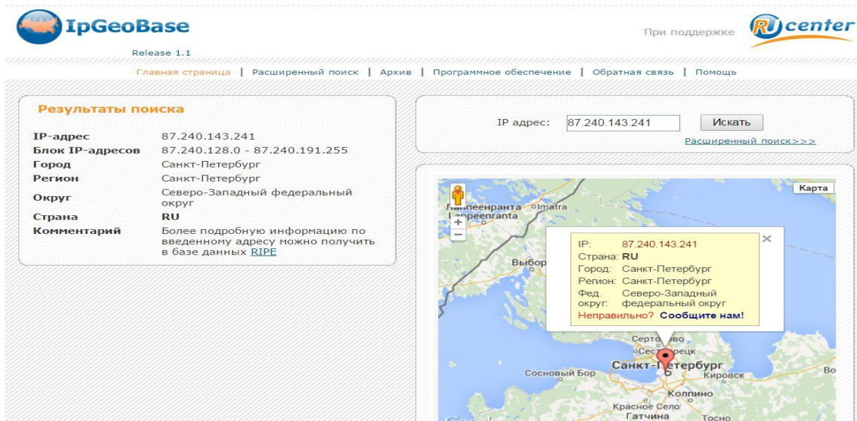
Рис. 4. Сервис Whois
