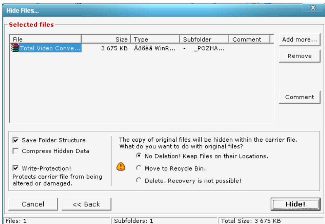
Рисунок 6 – Добавление файлов
