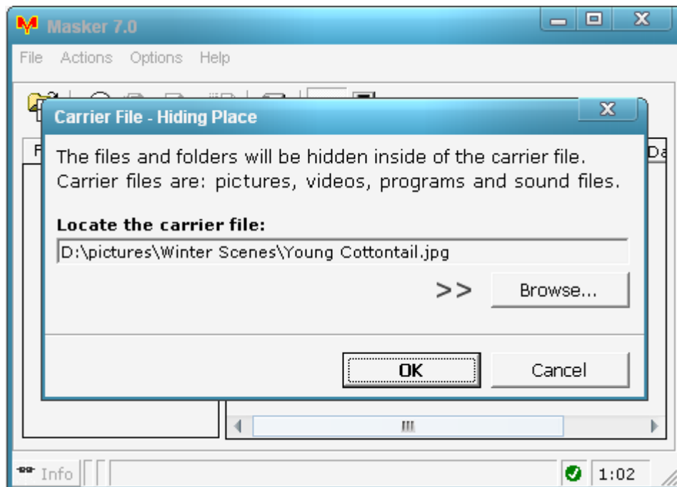
Рисунок 4 – Выбор файла-контейнера
