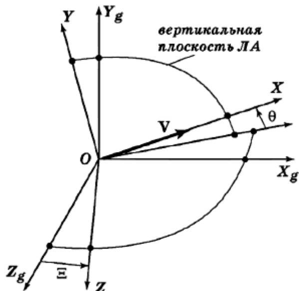
Рис. 4.4. Скоростная система координат: угол наклона траектории и путевой угол
