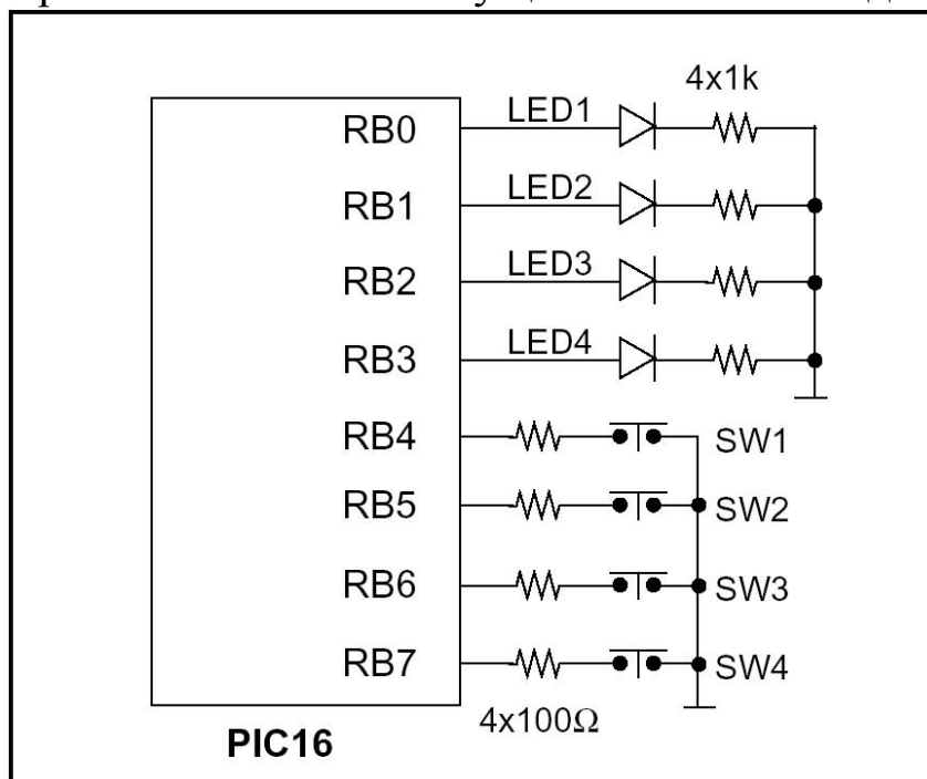
Рисунок 5.4 – Подключение клавиатуры для реализации низкопотребляющего режима работы микроконтроллера (sleep – режим) [Инструкция по применению AN552 - Microchip]
