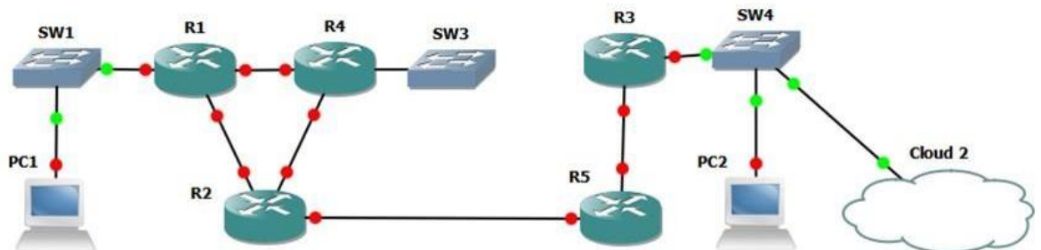
Рисунок 9 – Конфигурация моделируемой компьютерной сети
