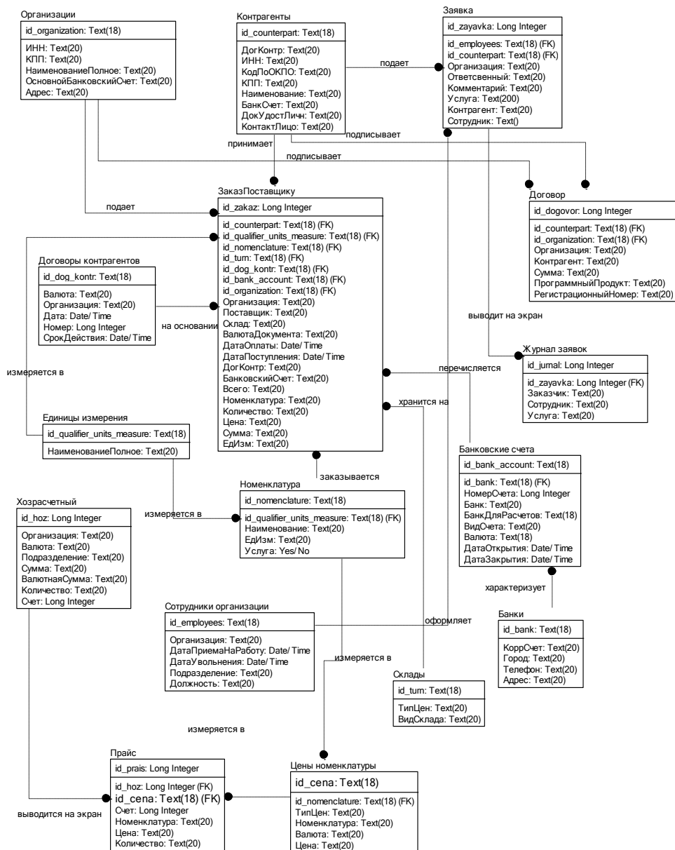
Рисунок 8 - Физическая модель БД
