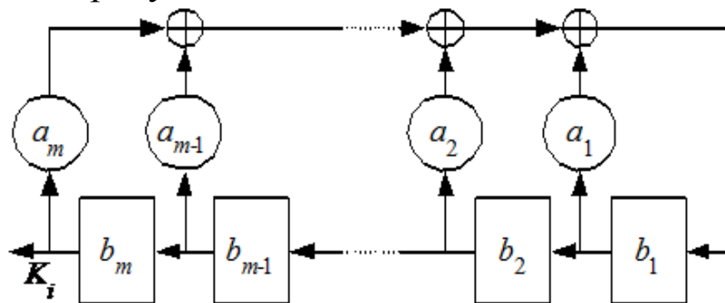
Рисунок 2 - Обобщенная схема LFSR
