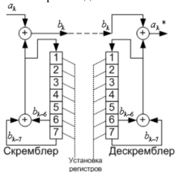
Рисунок 7 - Аддитивные скремблер и дескремблер
