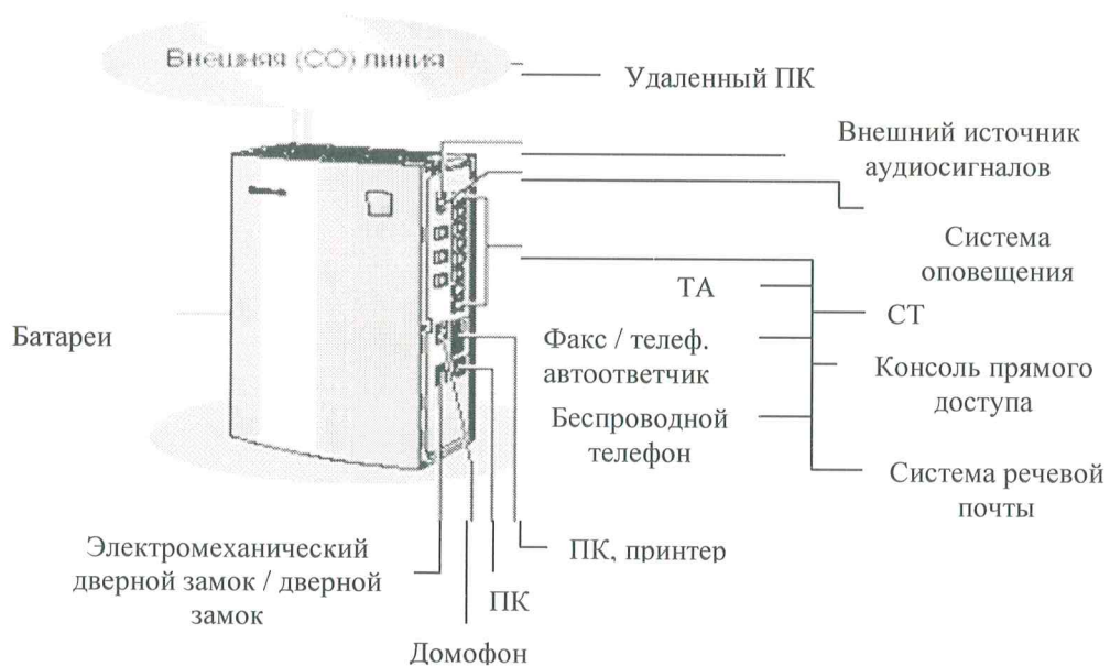
Рис. 1. Схема соединений в системе
