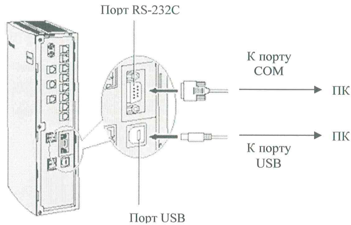
Рис. 4. Подключение ПК к портам УАТС
