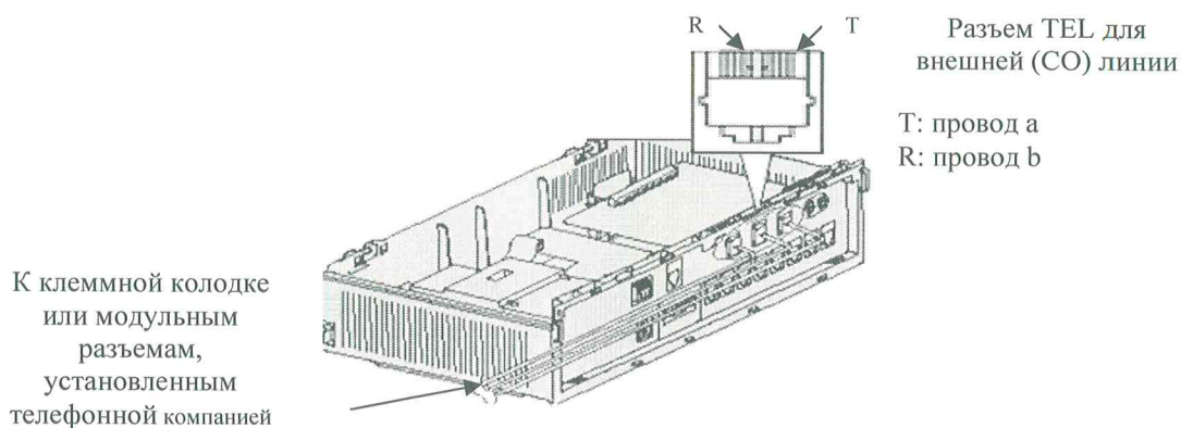
Рис. 2. Подключение соединительных проводов к клеммной колодке
