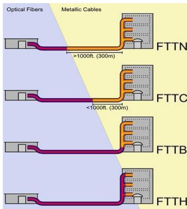
Рисунок 1 – Виды архитектуры FTТх
