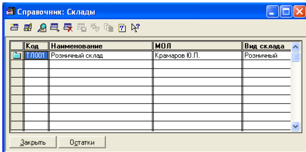
Рис. 1. Справочник Склады
