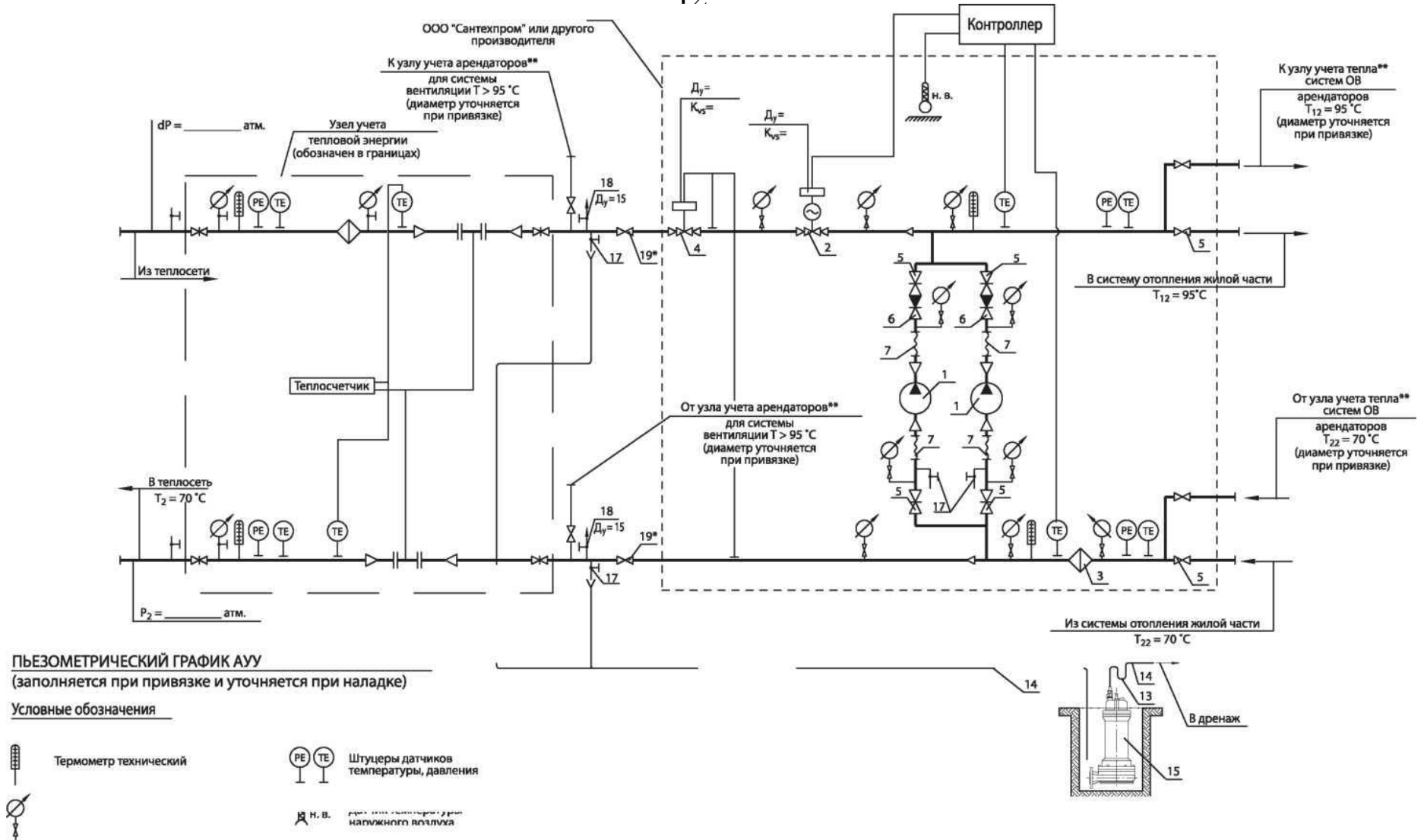
– Рис. 2 - Схема АУУ со смесительным насосом на перемычке между подающей и обратной магистралями.
