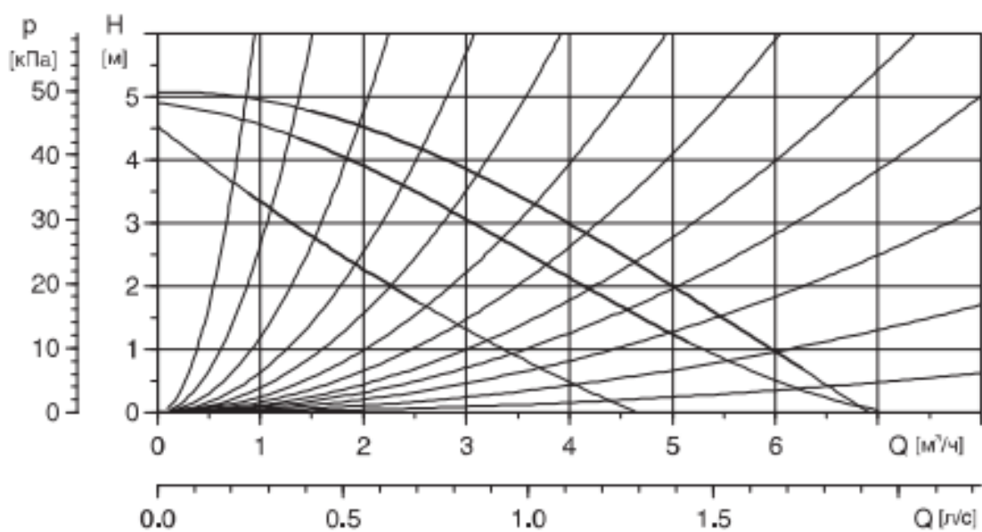
Рис.П. 4.7. Характеристики регулируемого электронасоса UPS 25-55
