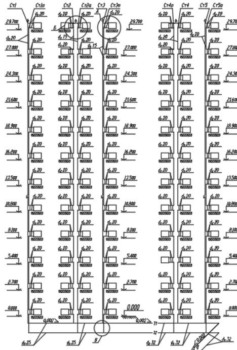
АксонOMETрическая схема системы отопления
