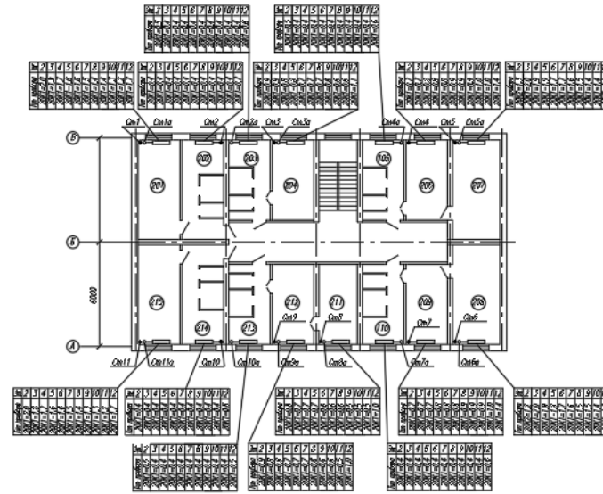
План типового этажа здания
