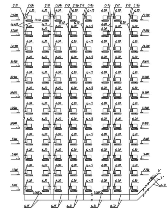
АксонOMETрическая схема системы отопления
