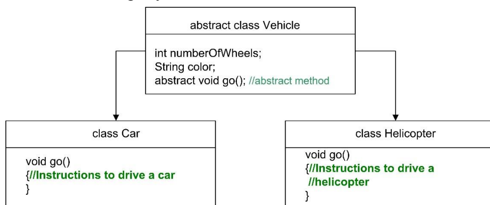
Рисунок 3.1. Иерархия классов
