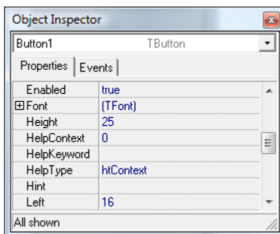
Рис. 2.6 Окно Object Inspector, отображающее свойства компонента Button
