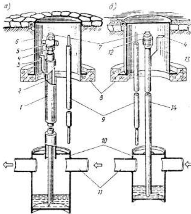
Рис.1 - Конденсатосборник
