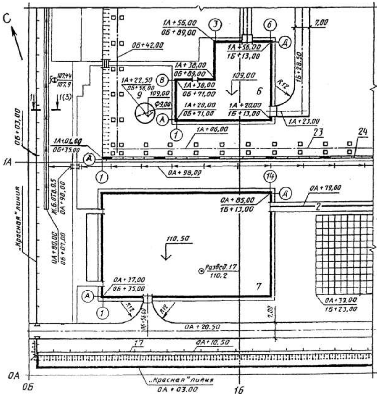
Рисунок 1 – Пример выполнения схемы планировочной организации земельного участка
