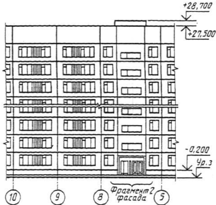
Рисунок 4 - Пример выполнения фасада жилого дома
