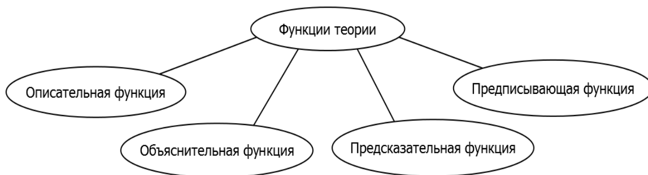
Рисунок 4. Функции теории
