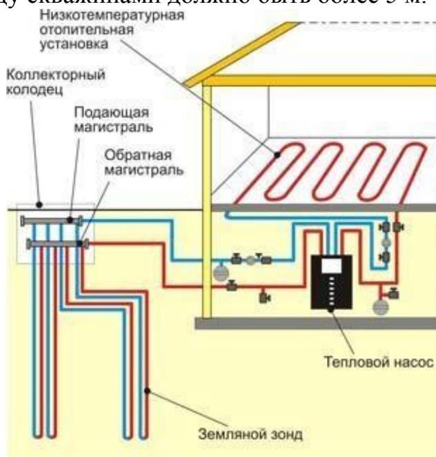
Рис. 7. Схема расположения земляного зонда
